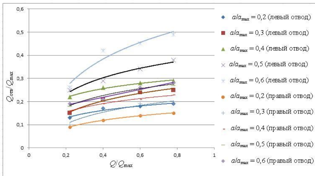
Рисунок 6 – Графики зависимости Q_{\text{отв}}/Q_{\max} = f(Q/Q_{\max})
