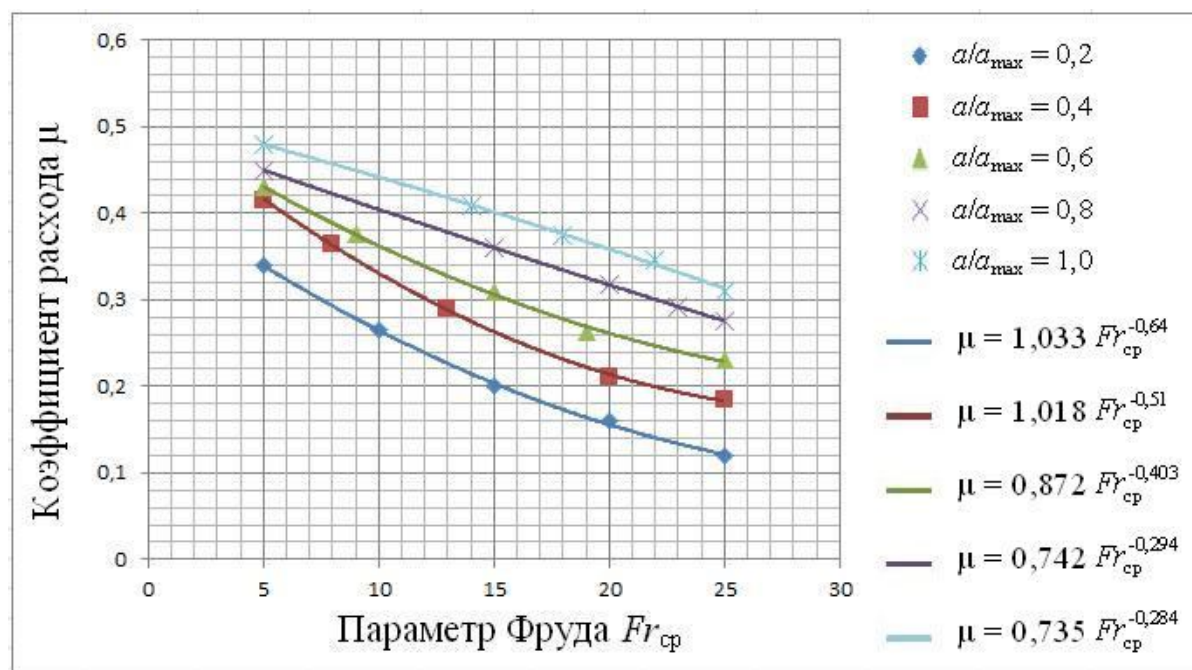
Рисунок 4 – Зависимость коэффициента расхода решетчатой плиты двухстороннего вододелителя от параметра Фруда \mu = f(Fr_{ср})
